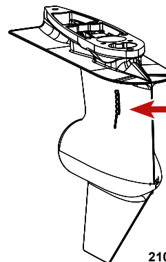
Seitlicher Wassereinlass
