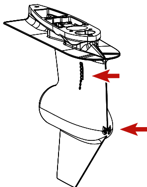
Doppelter Wassereinlass
